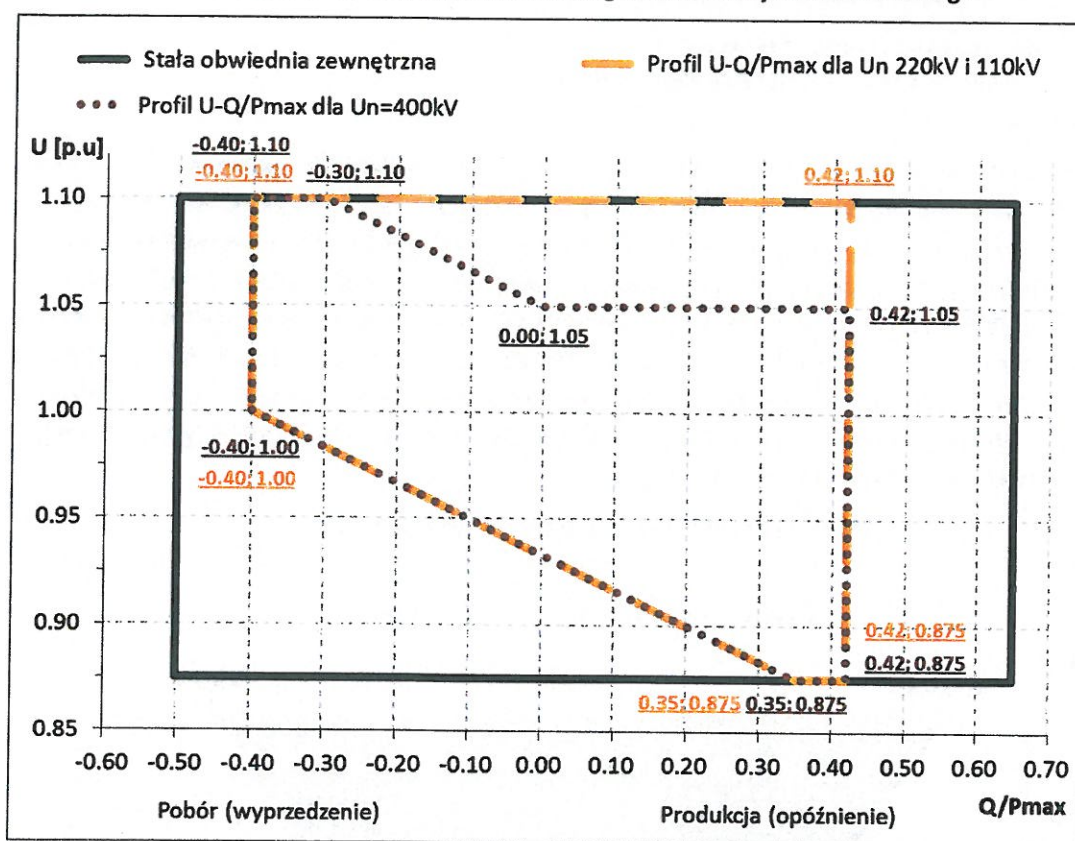
Profil U-Q/Pmax synchronicznego modułu wytwarzania energii
